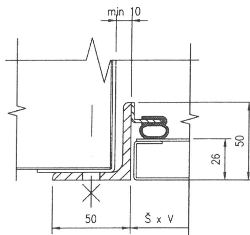
RÁM BEZ KOTEV S OTVORY
