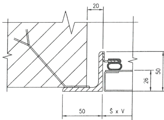
RÁM S KOTVAMI DO ZDIVA
